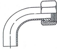
FGS90 FEMM A 90° . GIR. A SALDARE GAS
