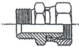
NMFG MASCH./FEMM. DIRITTO - GAS
