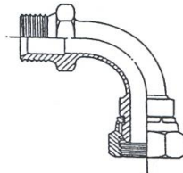
NMFG90 MASCH./FEMM. 90° - GAS
